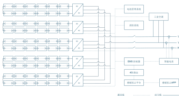
睿耐拓 ES1075 系统配置
